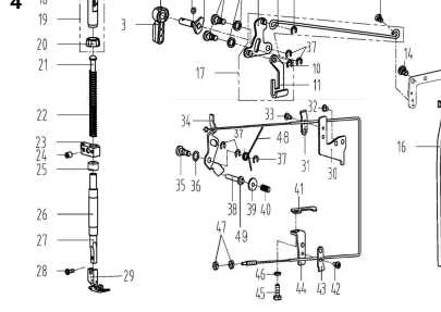
4. 压杆、自动抬压杆分组件/Presser Bar & Auto Lifter Components
